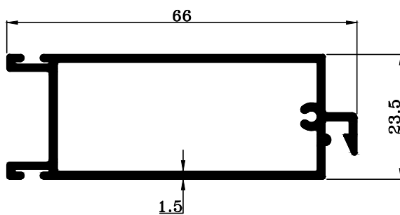
TRT-1447 W : 0.682 KG./M.
