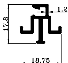
TRT-1451 W : 0.222 KG./M.
