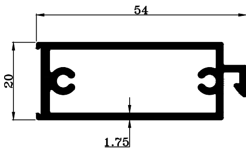
TRT-1446 W : 0.810 KG./M.
