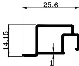
TRT-2000 W : 0.195 KG./M.
