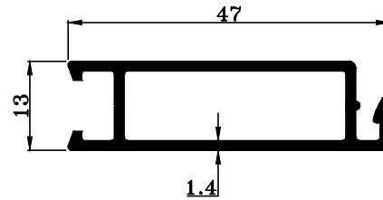
TRT-1444 W : 0.454 KG./M.
