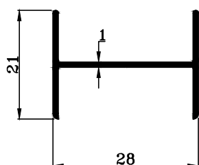
TRT-1450 W : 0.182 KG./M.
