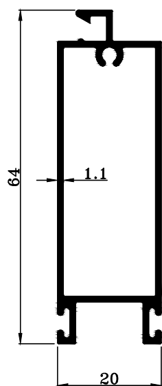
TRT-1448 W : 0.562 KG./M.
