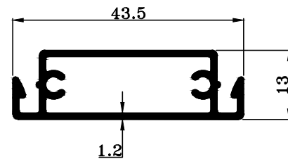
TRT-1445 W : 0.427 KG./M.
