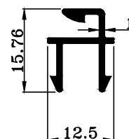
TRT-1452 W : 0.135 KG./M.
