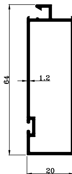
TRT-1449 W : 0.547 KG./M.
