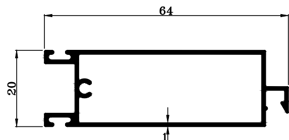
TRT-2939 W : 0.511 KG./M.
