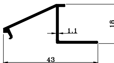
TRT-1109338 W : 0.215 KG./M.
