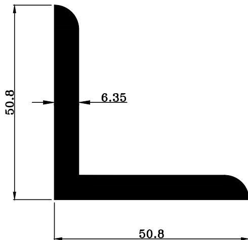
TRT-4437 W : 1.592 KG./M.
