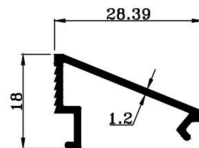
TRT-1209338 W : 0.196 KG./M.
