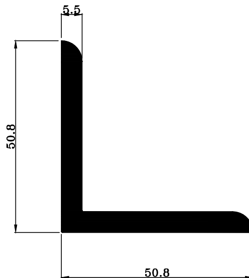
TRT-1200 W : 1.397 KG./M.
