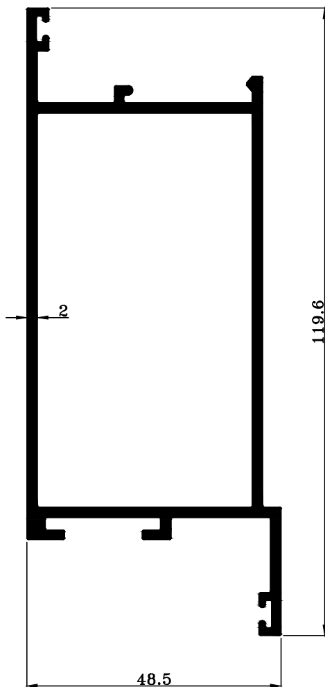
TRT-2009336 W : 1.734 KG./M.
