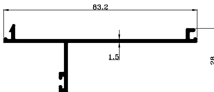
TRT-1503576 W : 0.516 KG./M.
