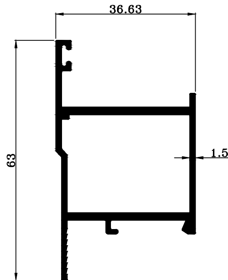
TRT-8912 W : 0.823 KG./M.
