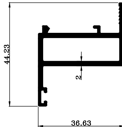
TRT-2004438 W : 0.715 KG./M.
