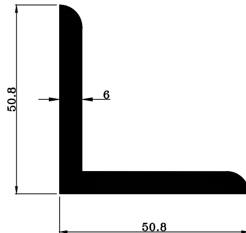
TRT-4438 W : 1.513 KG./M.
