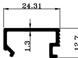
TRT-1303955 W : 0.193 KG./M.
