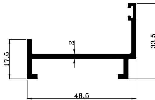
TRT-2009336 W : 0.548 KG./M.
