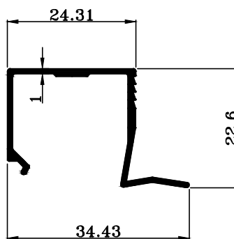
TRT-1003441 W : 0.238 KG./M.
