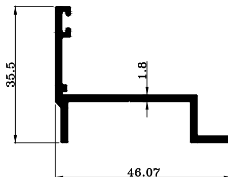
TRT-8913 W : 0.472 KG./M.
