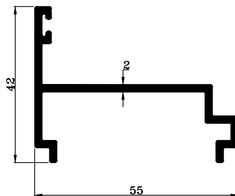
TRT-2009337 W : 0.696 KG./M.
