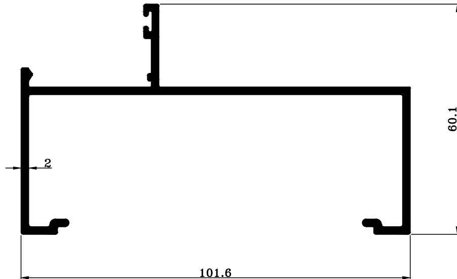
TRT-2003575 W : 1.252 KG./M.
