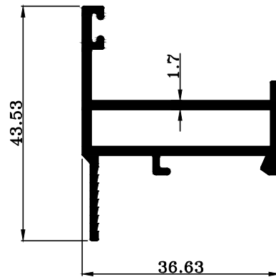
TRT-8911 W : 0.629 KG./M.
