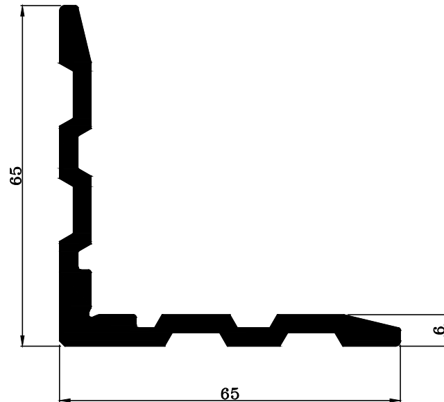
T 06011 W : 1.478 KG./M.
