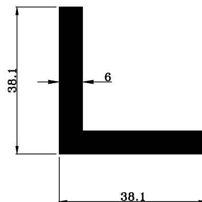
TRT-4440 W : 1.141 KG./M.
