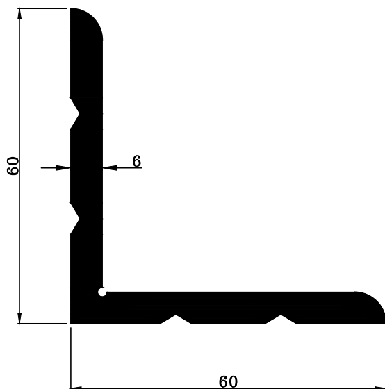
TRT-4439 W : 1.748 KG./M.
