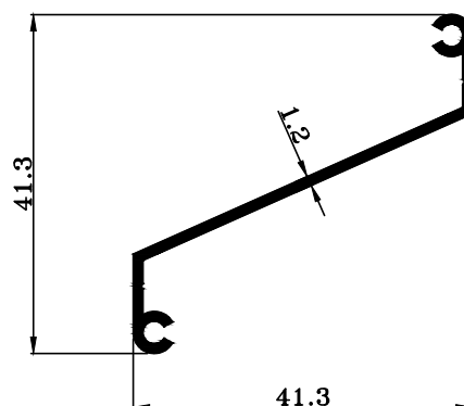
T 07003 W : 0.259 KG./M.
