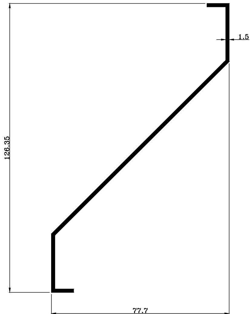
TRT-1417 W : 0.709 KG./M.
