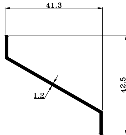
TRT-1425 W : 0.212 KG./M.
