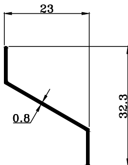
TRT-1428 W : 0.097 KG./M.
