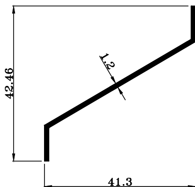
TRT-1412 W : 0.213 KG./M.
