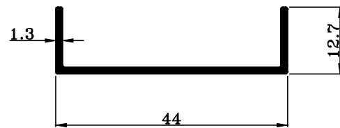
TRT-1426 W : 0.234 KG./M.
