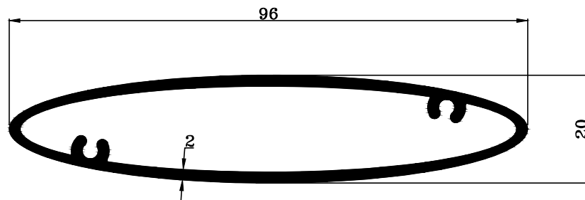
TRT-1432 W : 1.137 KG./M.
