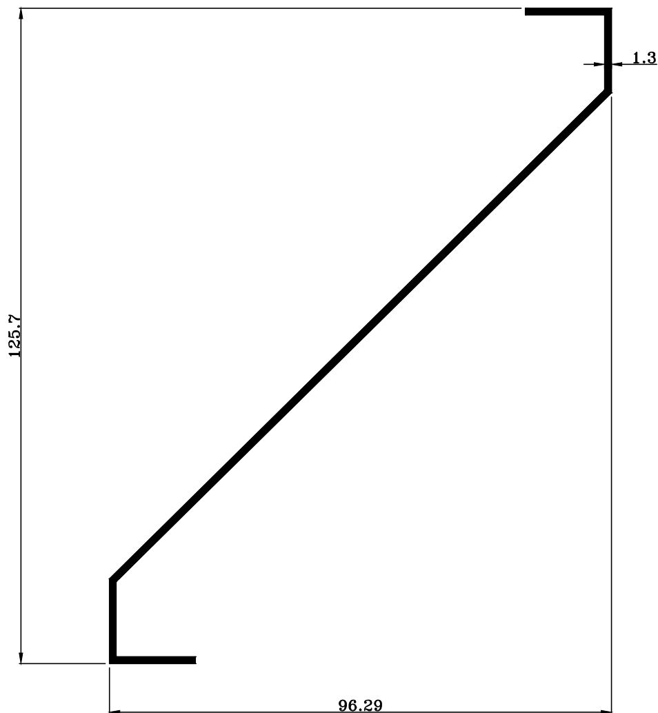
TRT-1421 W : 0.690 KG./M.
