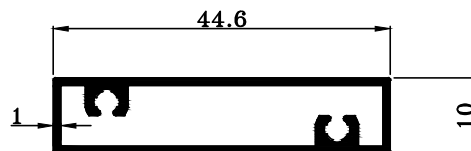
T 06027 W : 0.358 KG./M.
