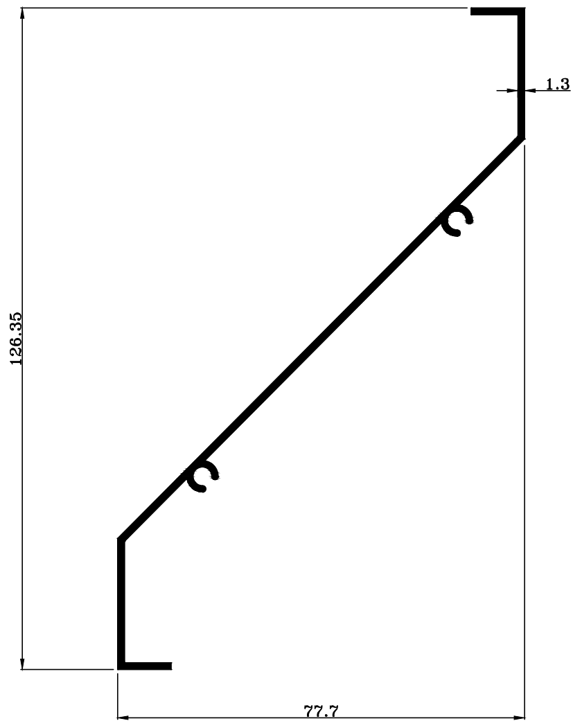
TRT-1419 W : 0.677 KG./M.
