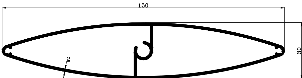
TRT-1434 W : 1.438 KG./M.
