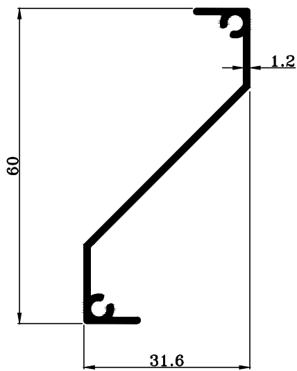
T 15006 W : 0.334 KG./M.
