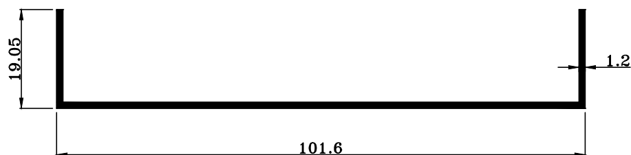
TRT-1422 W : 0.4446 KG./M.
