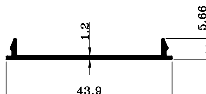
T 06029 W : 0.169 KG./M.
