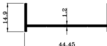
TRT-1414 W : 0.233 KG./M.
