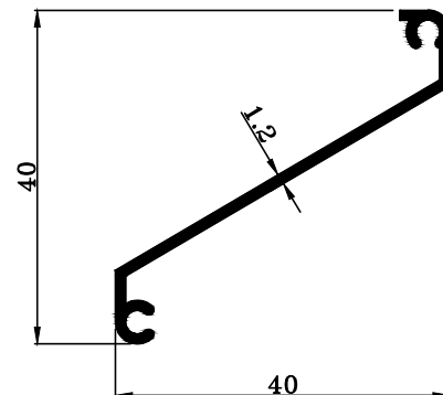
TRT-1411 W : 0.248 KG./M.
