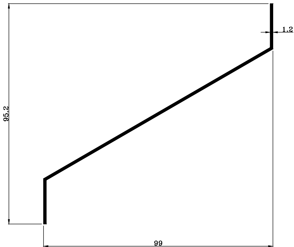
TRT-1423 W : 0.493 KG./M.
