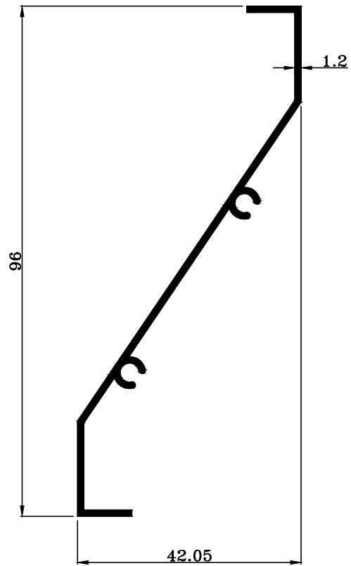
TRT-1415 W : 0.470 KG./M.
