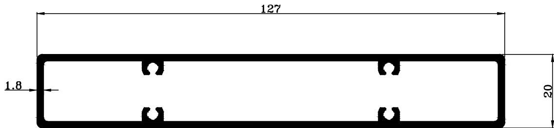
T 06023 W : 1.520 KG./M.
