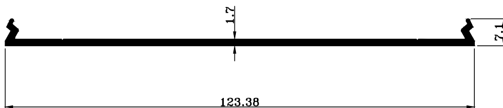
T 06026 W : 0.651 KG./M.
