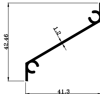
TRT-1413 W : 0.270 KG./M.
