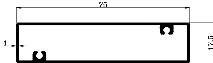
T 06024 W : 0.560 KG./M.
