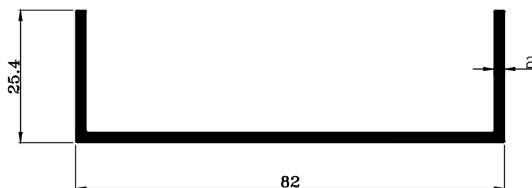
TRT-1416 W : 0.698 KG./M.
