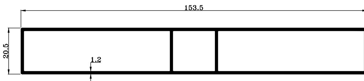
TRT-1438 W : 1.229 KG./M.
