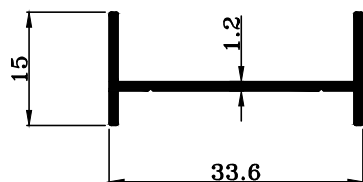
T 15005 W : 0.198 KG./M.
