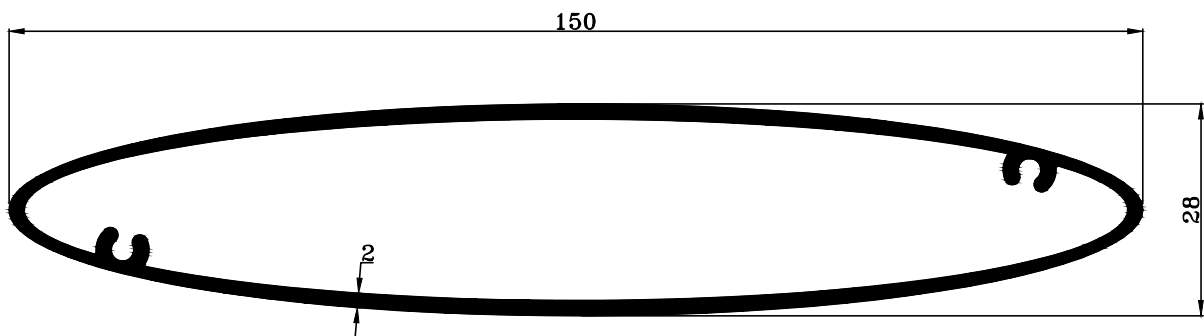
TRT-1433 W : 1.753 KG./M.
