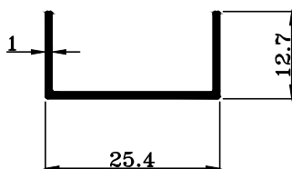
TRT-1429 W : 0.131 KG./M.
