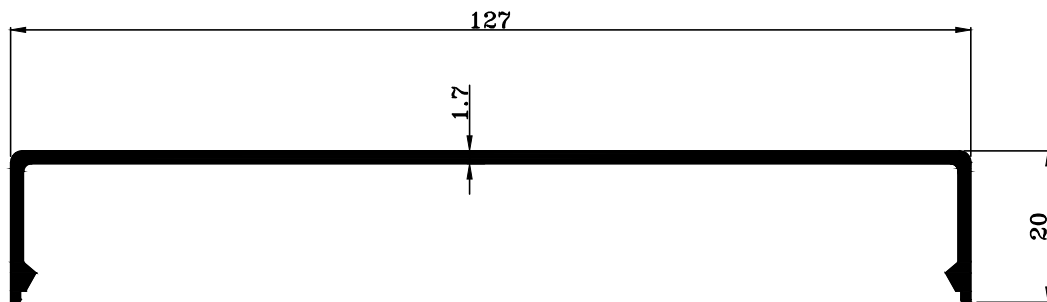
T 06025 W : 0.765 KG./M.
