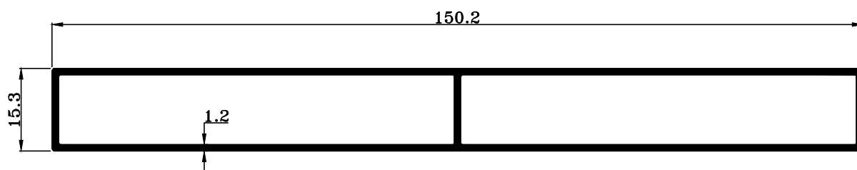
TRT-1437 W : 1.098 KG./M.
