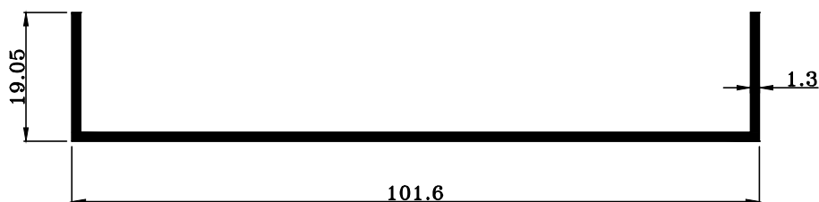
TRT-1420 W : 0.483 KG./M.
