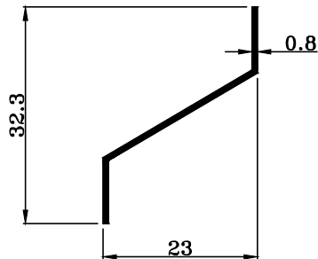
TRT-1410 W : 0.098 KG./M.
