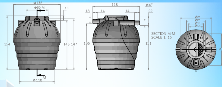
TREATMENTTANK (ZAD) - 1600L.
