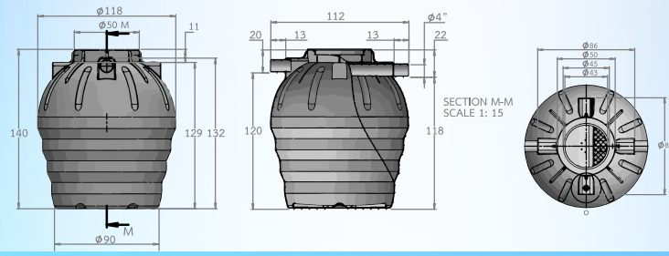
TREATMENTTANK (ZAD) - 1600L.
