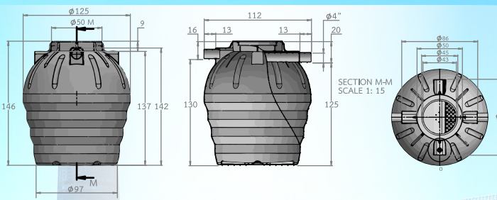
TREATMENTTANK (ZAD) - 1200L.
